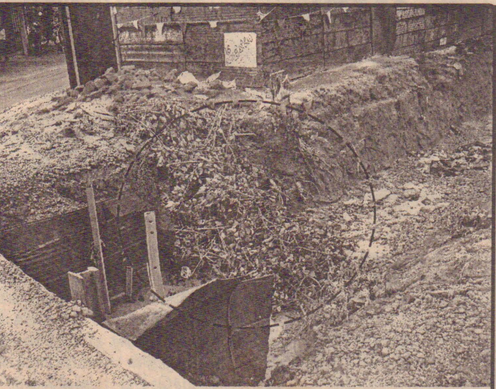
புதுக்குடியிருப்பு மாத்நளன் வீதியில் நீர் செல்வதற்காக வீதியின் இருமருங்கிலும் வடிகால் வெட்டப்பட்டுள்ளது. இவ்வடிகால்களில் நீர் செல்லாது குப்பை போடப்பட்டுள்ளதை படத்தில் காணலாம். (படம்: தவரட்சன்)
