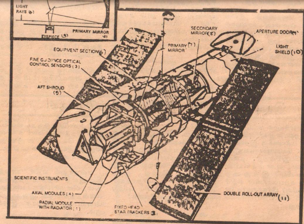
(1) கதிர்வீச்சு தடைகருவி (Radial module with radiator) (2) விண்விம்பங்கள் இனங்காணுகருவி (Fixed Head star Trackers) (3) ஒளிக்கதிர்களை கட்டுப்படுத்தும் கருவி (Fine Guidance optical control sensors) (4) அச்சு கட்டுப்படுத்தி (Axial modules) (5) பாதுகாப்பு உடல் (Aft Shroud) (6) தொடர்பு இயக்கப்பகுதி (Equipment section) (7) முதன்மை ஆடி (Primary mirror) (8) விம்பம் எதிரொளிக்கும் ஆடி (Secondary mirror) (9) ஒளிபுகுவிடும் கதவு (Aperture Door) (10) ஒளிபுகுவிடும் தட்டு (Light Shield) (11) சூரியகலத்தட்டு (Double control outray)
